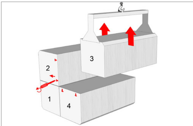
Bild 2: Gewindeschrauben entfernen
