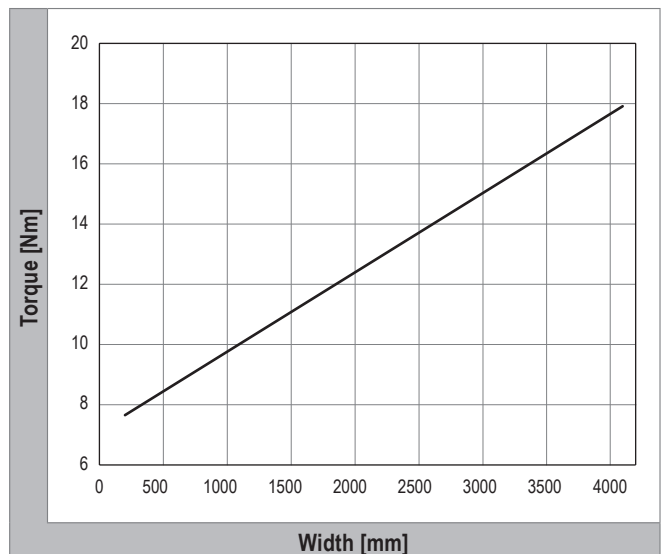
Fig. G5: Necessary torque per actuator
